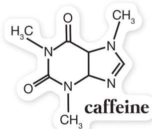
3-200303 CAFFEINE MOLECULE
